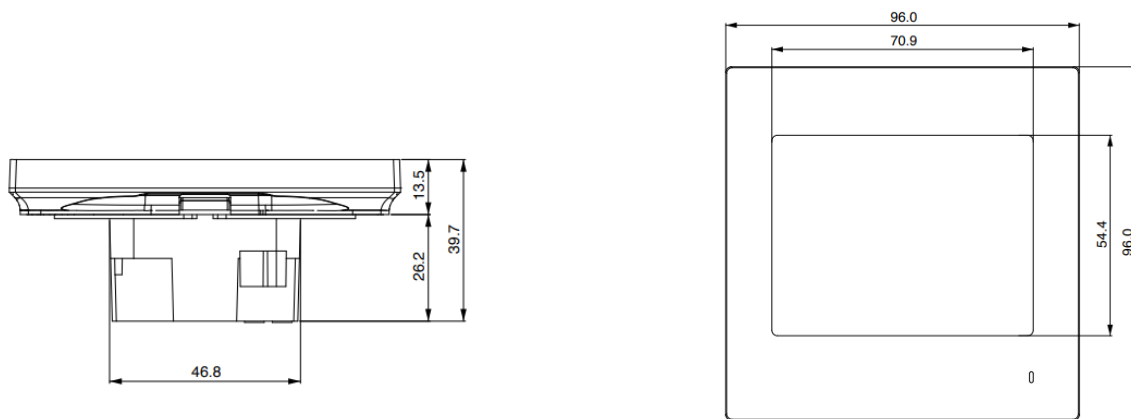
Abbildung 1: Abmessungen (mm) GRTP35
